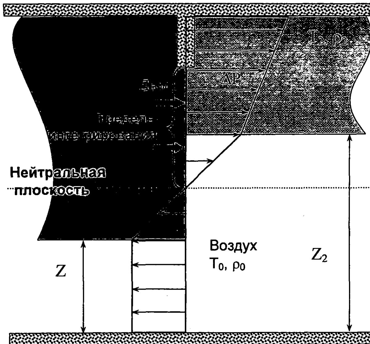
Рис. П6.1. Массопотоки через проем
