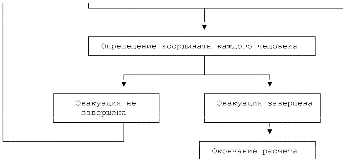
Рис. П3.2. Блок-схема определения расчетного времени эвакуации людей из здания
